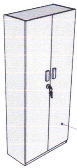
ARMARIO PERSPECTIVA ESCALA 1:25
