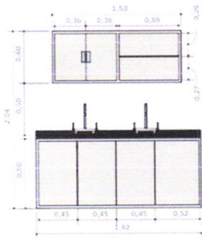
ARMÁRIO COZINHA VISTA LATERAL ESCALA 1:20
