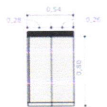
ARMÁRIO COZINHA VISTA LATERAL ESCALA 1:20
