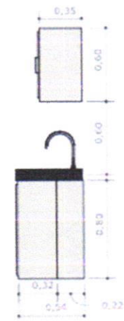
ARMÁRIO COZINHA VISTA LATERAL ESCALA 1:20
