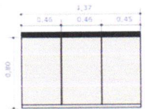
ARMÁRIO COZINHA VISTA LATERAL ESCALA 1:20
