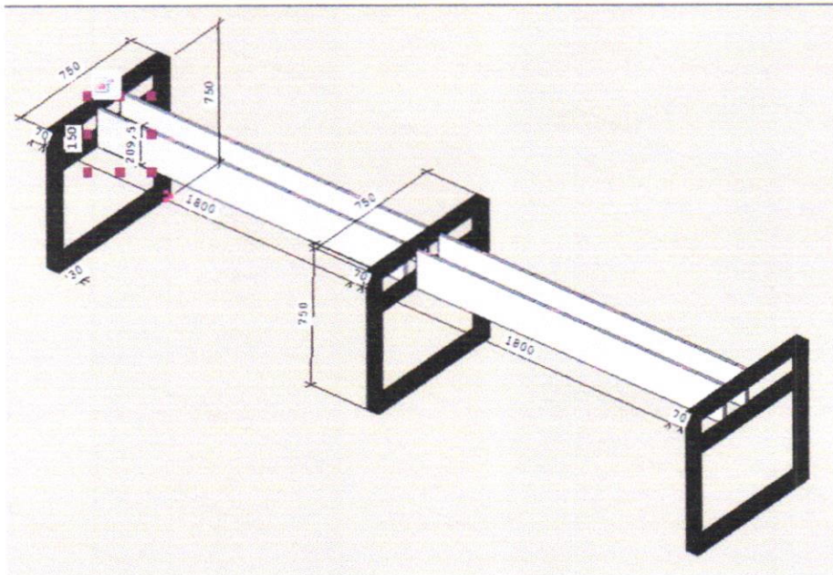
Base metálica para mesa de reunião, pintura preto fosco
