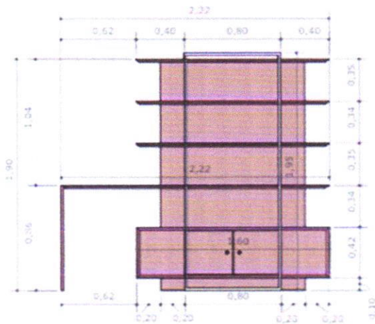
ARMÁRIO DO GABINETE VISTA FRONTAL ESCALA 1:20
