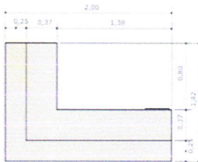
ANEXO 03 - SEÇÃO FRONTAL DA ESQUA - 1/20
