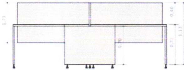
MESA COMPARTILHADA MDF MILANO LATA 1,20
