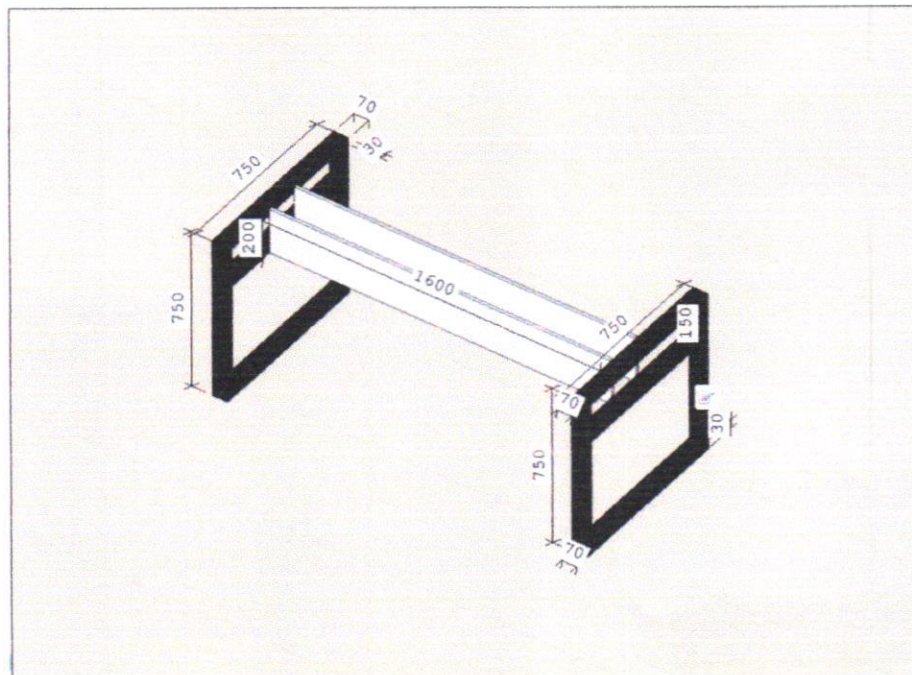
Base metálica para mesa do gabinete do prefeito, pintura preto fosco.
